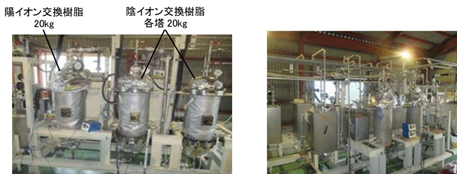
図1 完成した装置の写真(左:燃料製造装置、右:樹脂再生装置)
